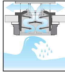
Válvula respiradero de bola flotante
